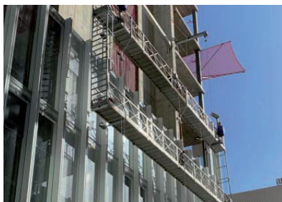
Doppelstöckige Seilarbeitsbühne zur Fassadenmontage
